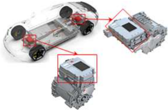
전력변환장치(인버터) 소프트웨어
