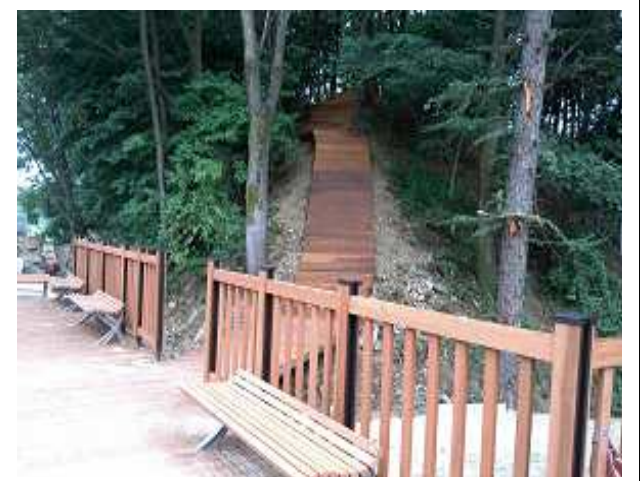
경부선 옥천쉼터(부산) : 낮은 절토부 산책로 조성
